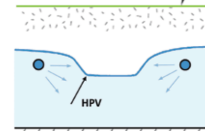
Obr. 3) Tři základní typy drenážních systémů: tradiční jedno-funkční drenáž; drenáž s regulovaným odtokem; regulační drenáž. Zdroj: Field Drainage Association; upravil Z. Kulhavý.
